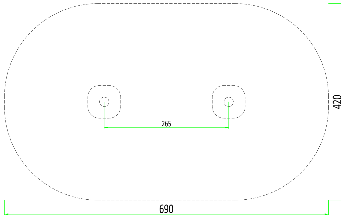
Draufsicht
