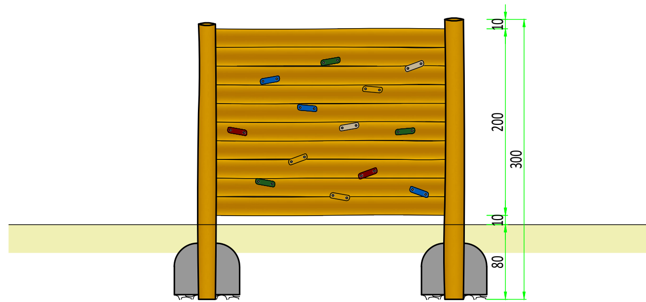
Ansichten
