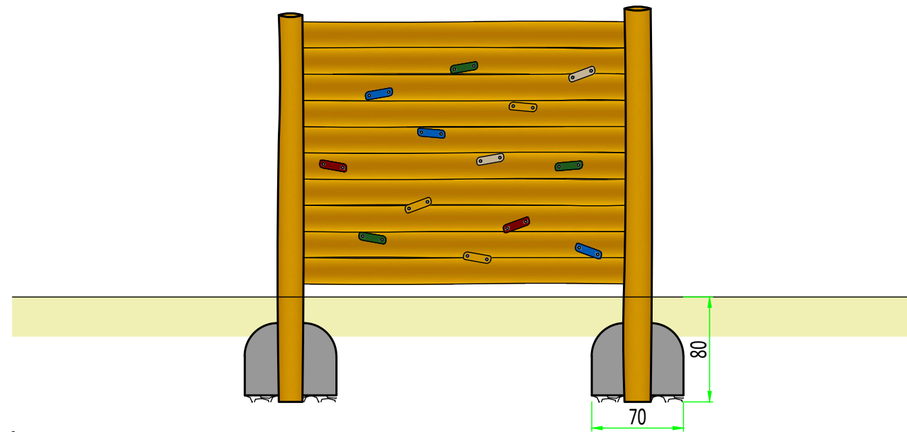
Ansichten
